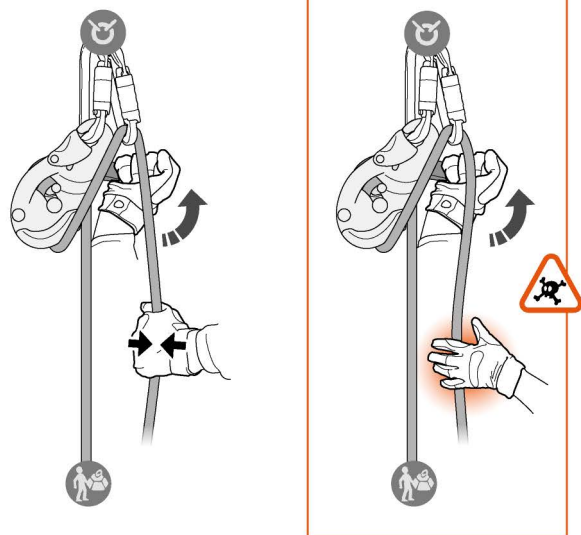
11a. Lowering Faire descendre
