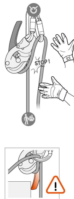
11c. Stop position Position d'arrêt
